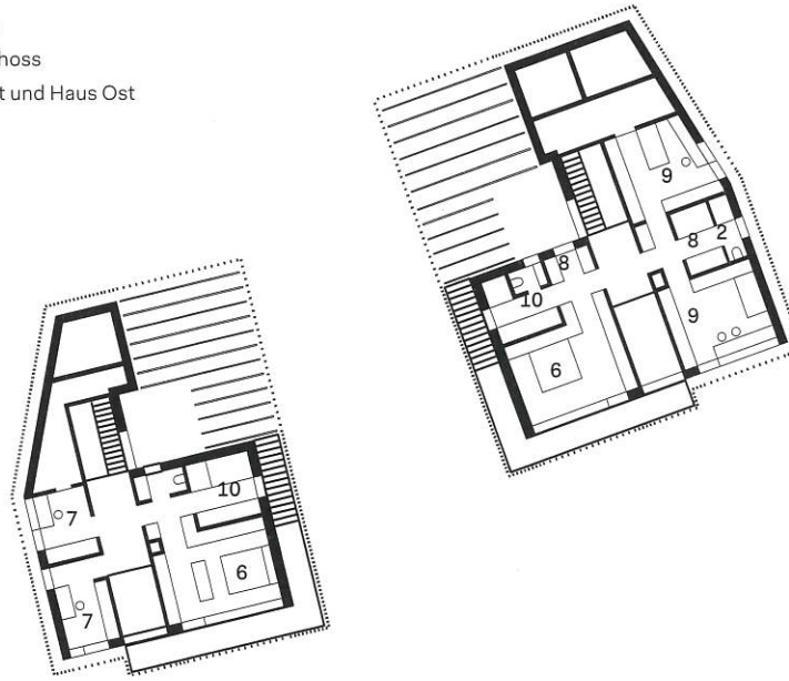
Grundriss
